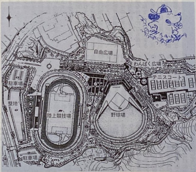
三原運動公園計画平面図
