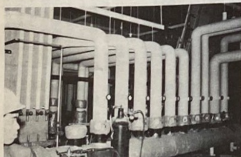
▲帝人からパイプラインで送られてくる水蒸気を 冷暖房と温水プールの熱源として活用する
